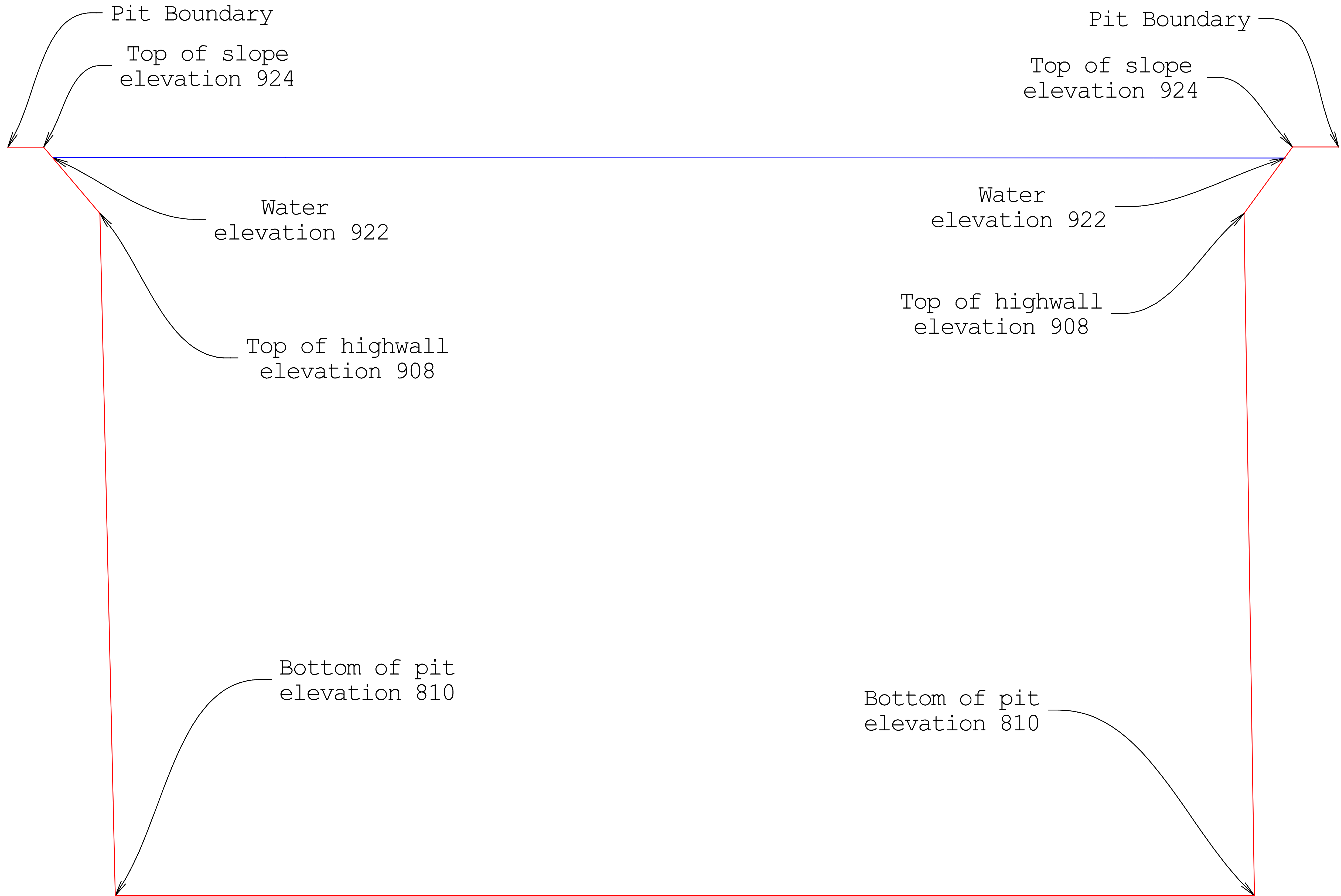
Cadott XX pit Cross section A-B
